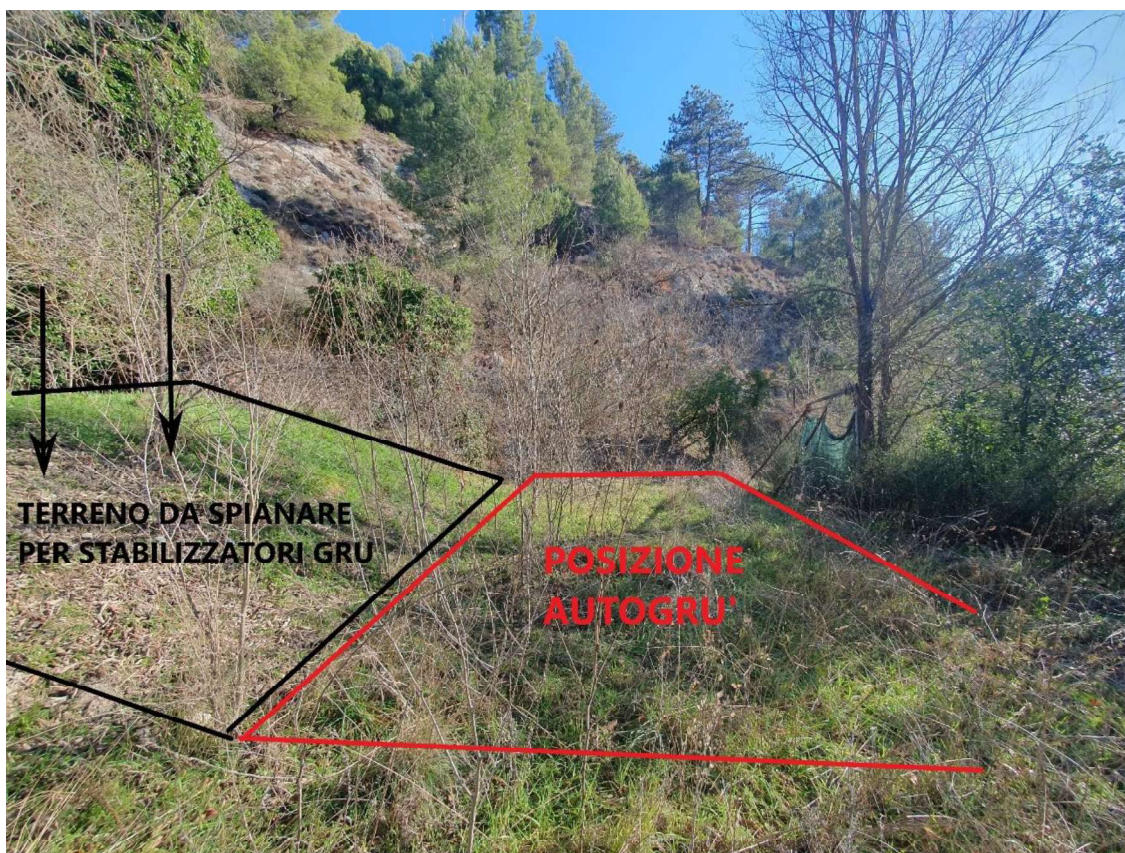
Foto n° 8 Posizionamento autogrù con terreno da spianare per gli stabilizzatori
